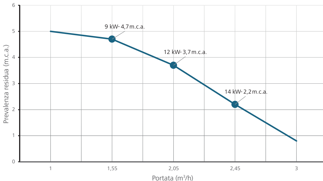
Diagrammi portata nominale/prevalenza residua circolatori
