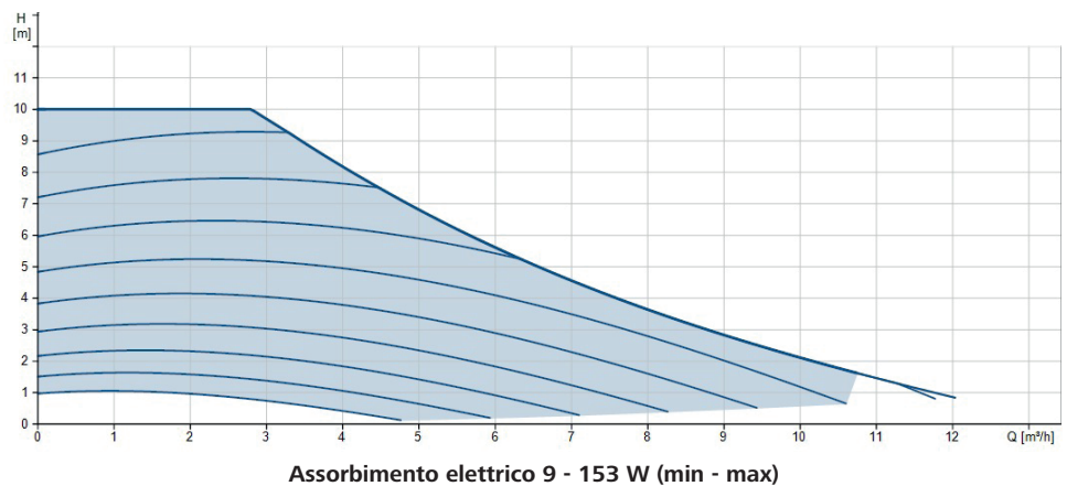
MAGNA 3 25-100
