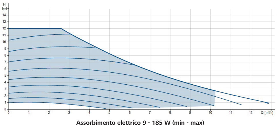
MAGNA 3 25-120
