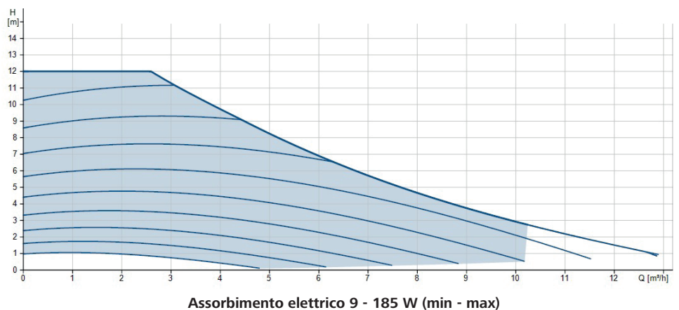
MAGNA 3 25-120
