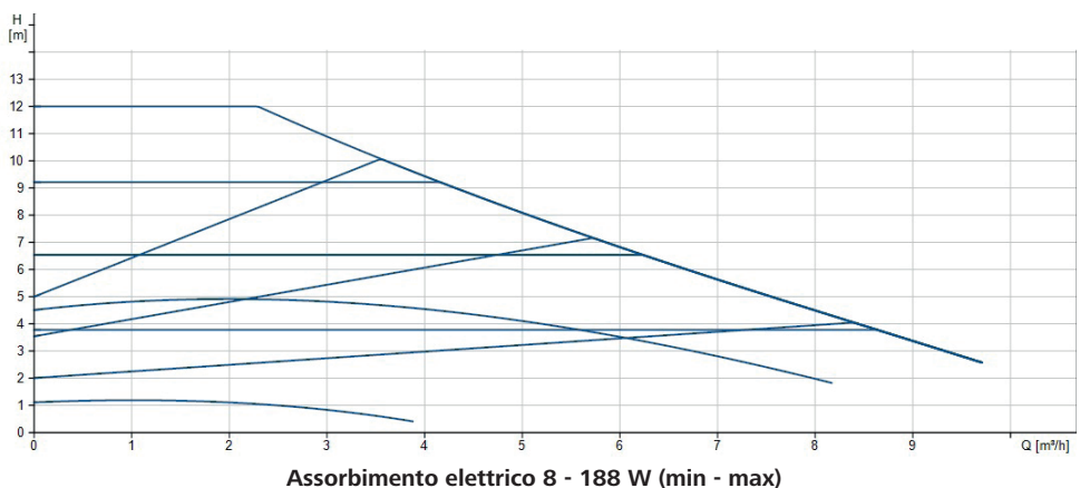
MAGNA 1 25-120
