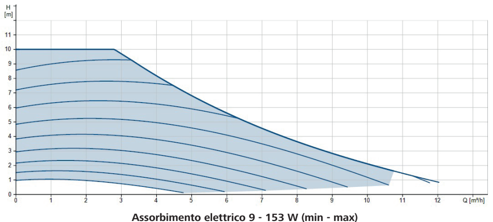
MAGNA 3 25-100
