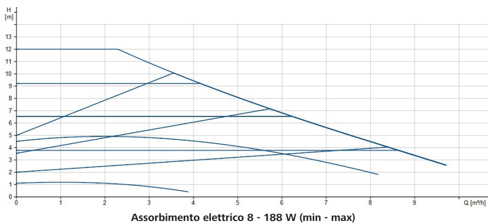
MAGNA 1 25-120
