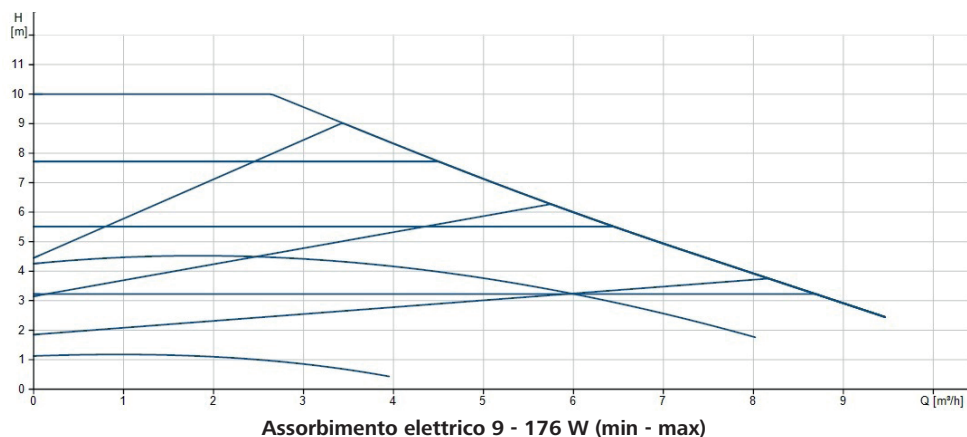
MAGNA 1 25-100
