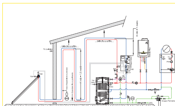
Impianto solare sottotetto con AquaSun Plus
