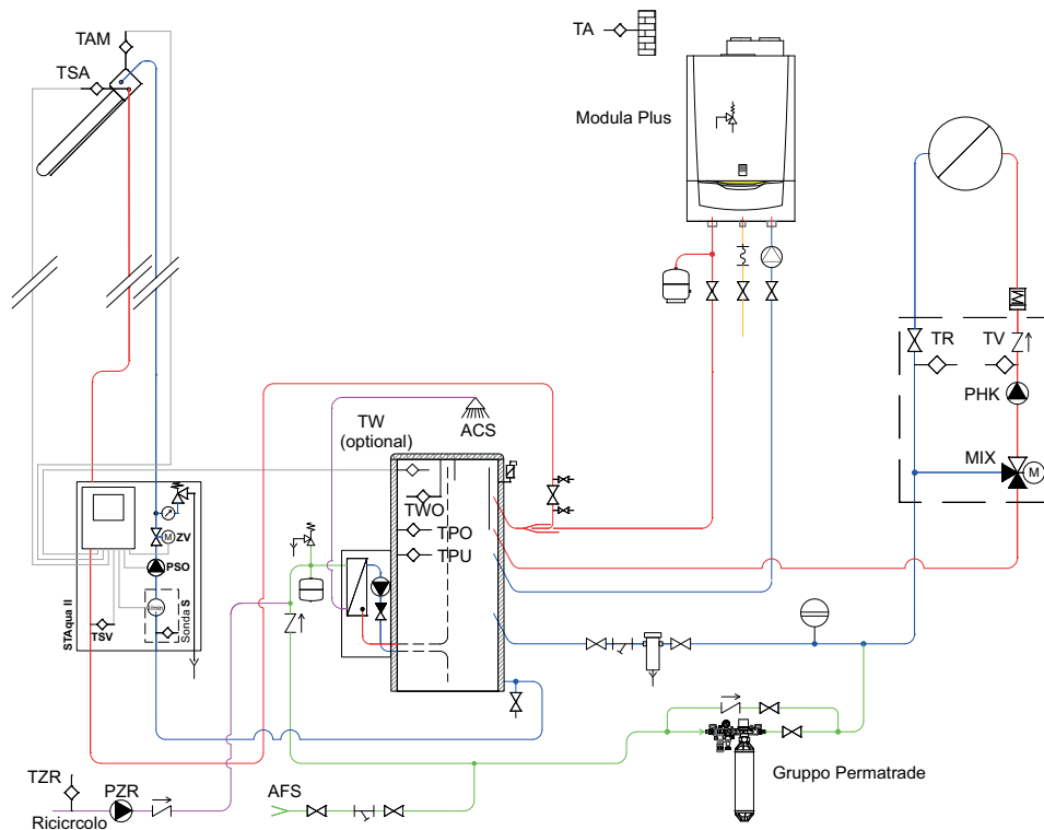
Pacchetti solari con AQUA EXPRESSO III per produzione acqua calda sanitaria e integrazione al riscaldamento (THIT2003)
