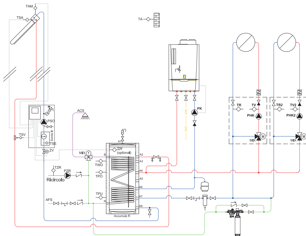
Pacchetti solari con bollitore combinato TITAN P-S per produzione acqua calda sanitaria e integrazione al riscaldamento (THIT9304)
