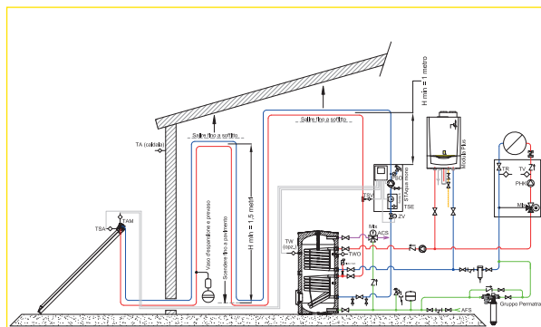
Impianto solare sottotetto con AquaSun Plus (solare su serpentina separata)
