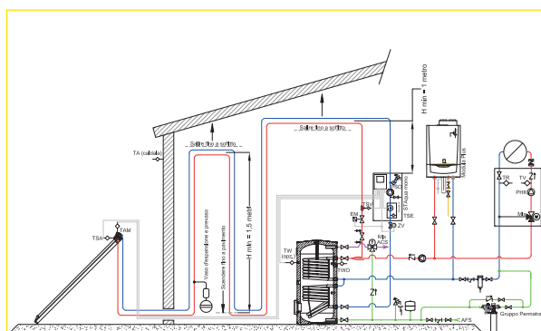
Impianto solare sottotetto con AquaSun Plus
