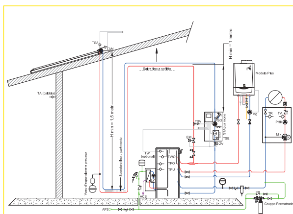
Impianto solare sottotetto con AQUA EXPRESSO III
