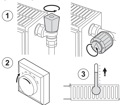
Fig.13 Degasare l'impianto
