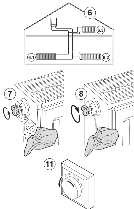
Fig.15 Degasare l'impianto
