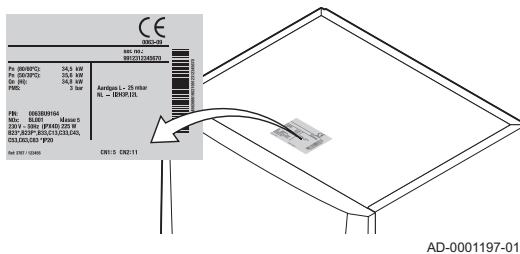
Fig.17 Targa matricola
