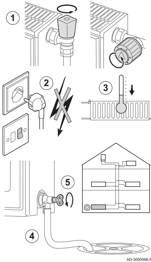
Fig.16 Svuotamento dell'impianto
