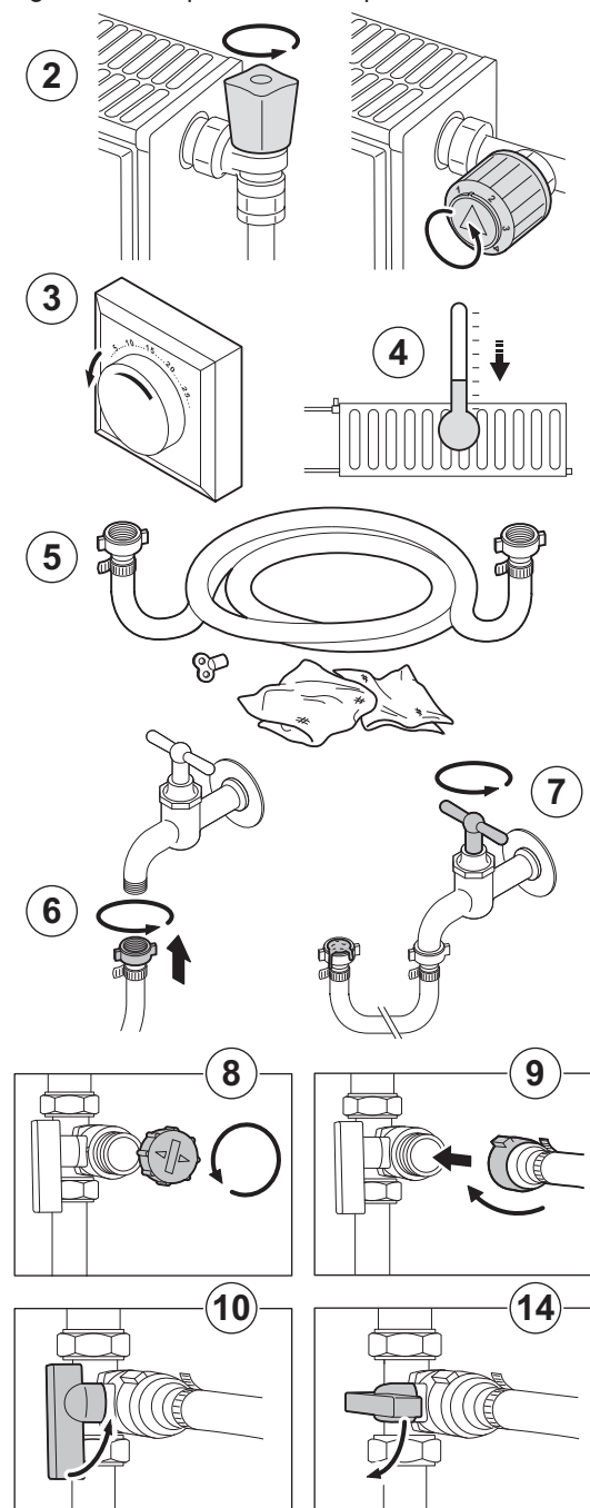
Fig.12 Riempimento dell'impianto
