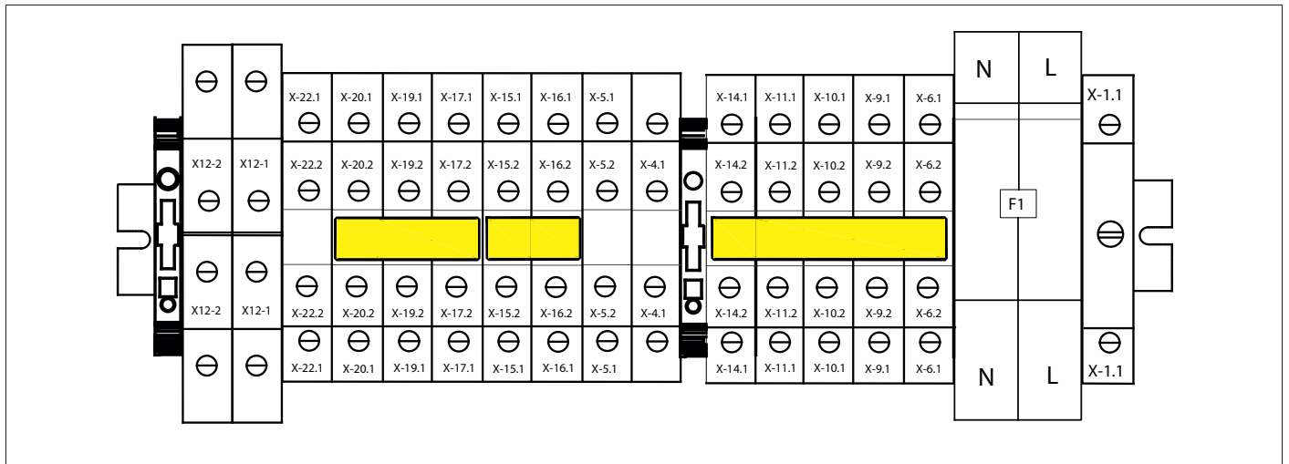
Morsettiera ModuExpo LT-06A MNSKAI32 / LT-10 MNSKAI32 / LT-12 MNSKAI32 (1ph)
