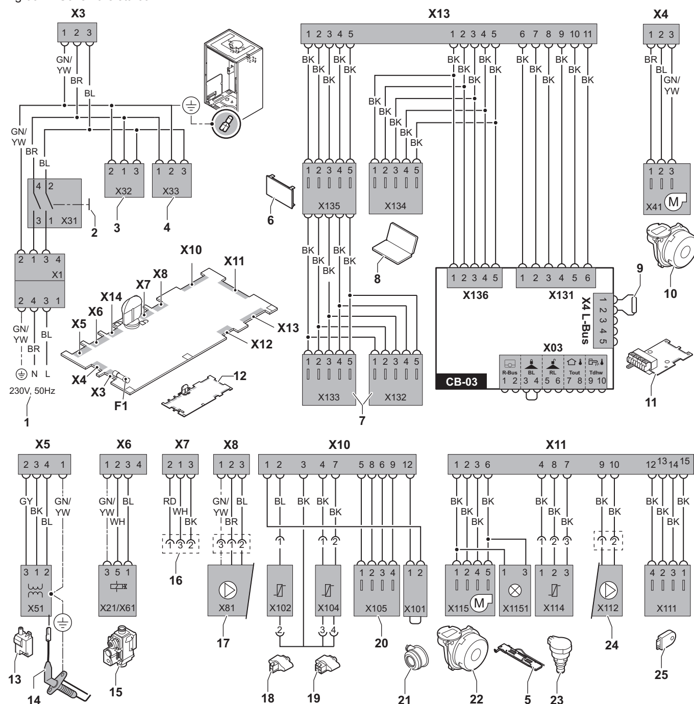
Fig.65 Schema elettrico
