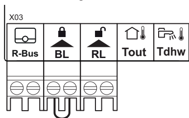
Fig.22 Connettori sulla PCB di collegamento
