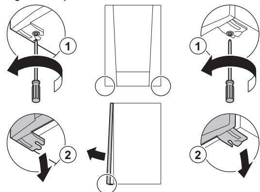
Fig.51 Apertura della caldaia
