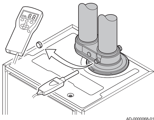
Fig.39 Presa analisi gas di scarico
