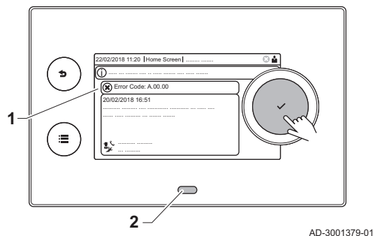
Fig.53 Visualizzazione del codice anomalia su HMI T-control
