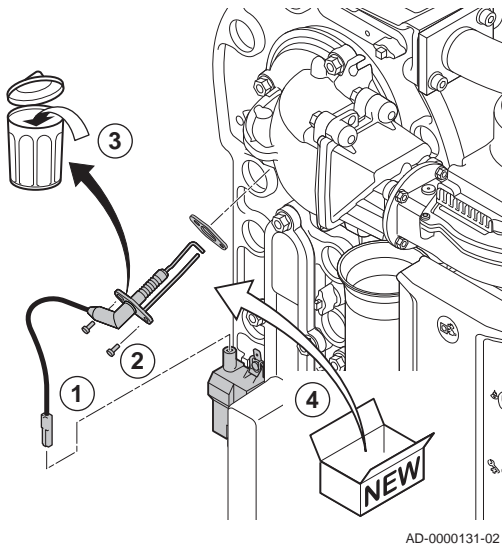
Fig.38 Sostituzione dell'elettrodo di accensione/ionizzazione
