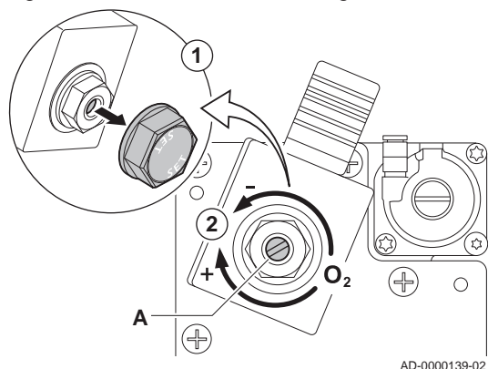
Fig.28 Posizione della vite di regolazione A
