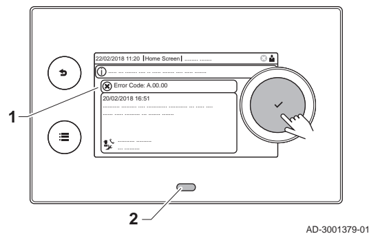
Fig.40 Visualizzazione del codice anomalia su HMI T-control
