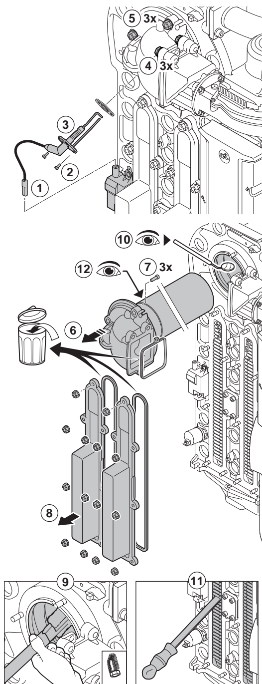
Fig.34 Controllo del bruciatore
