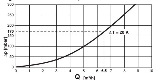
Fig.1 Resistenza acqua
