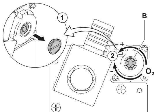
Fig.30 Posizione della vite di regolazione B
