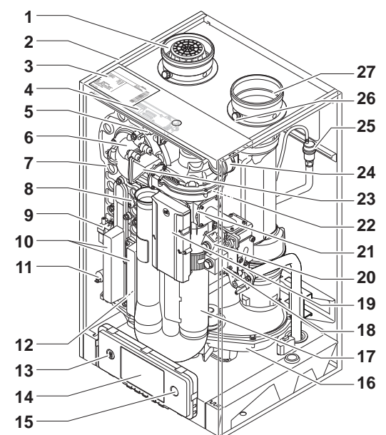
Fig.2 Componenti principali
