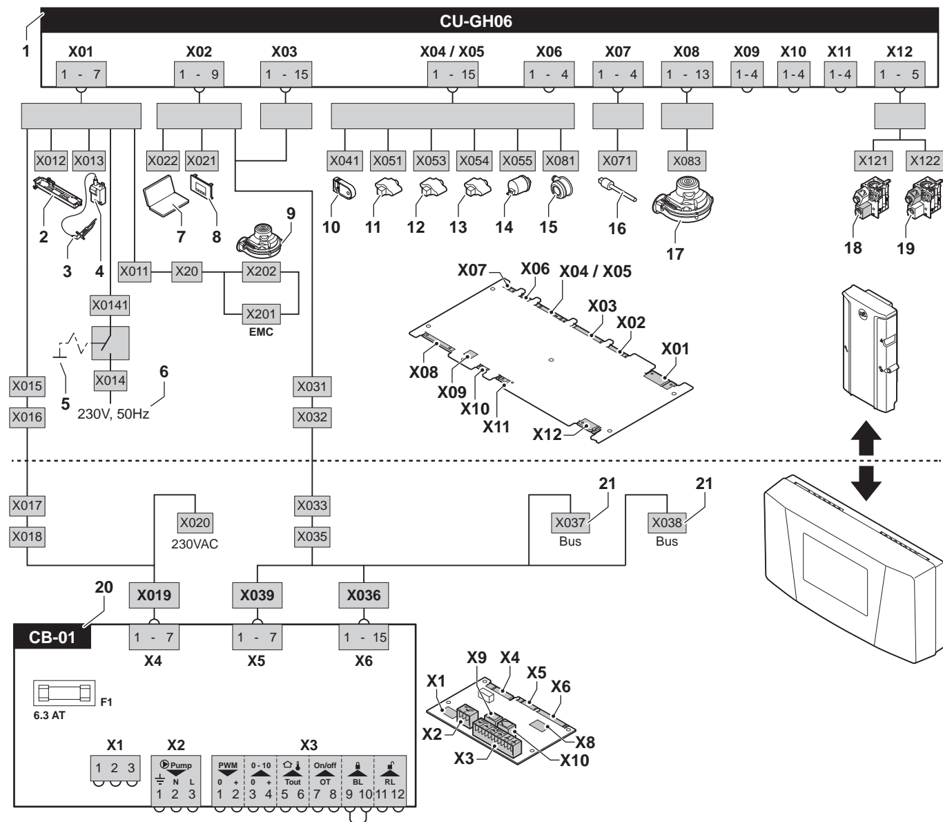
Fig.42 Schema elettrico
