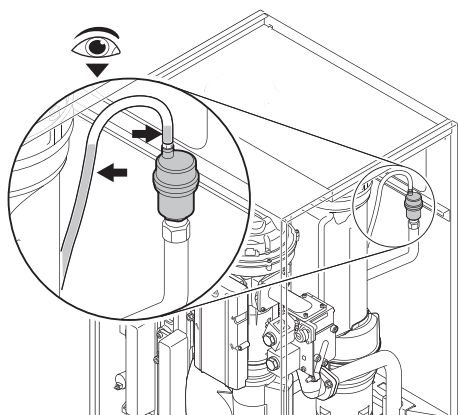
Fig.33 Controllo dello sfiato automatico
