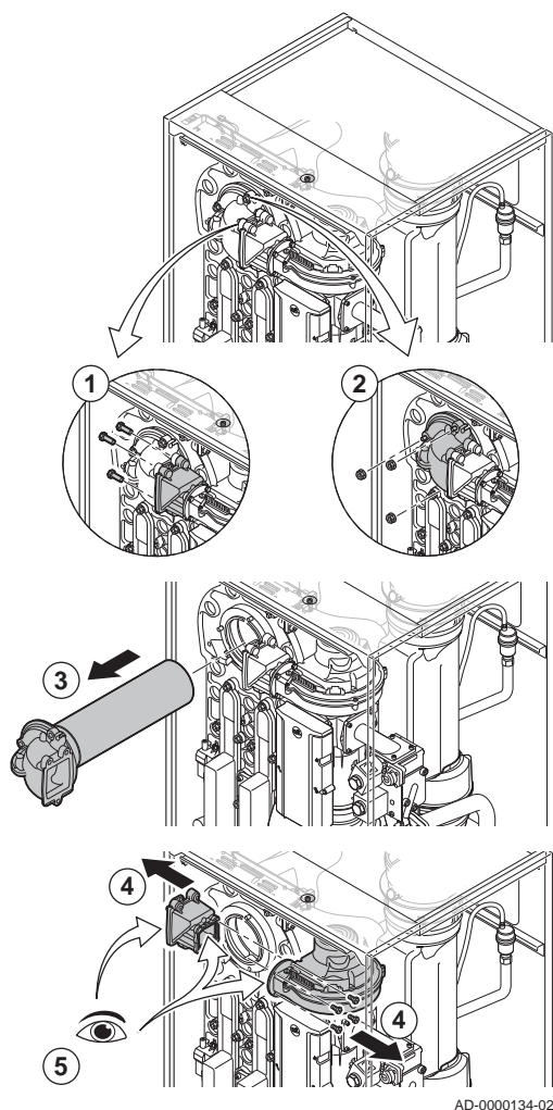
Fig.39 Controllo della valvola di non ritorno
