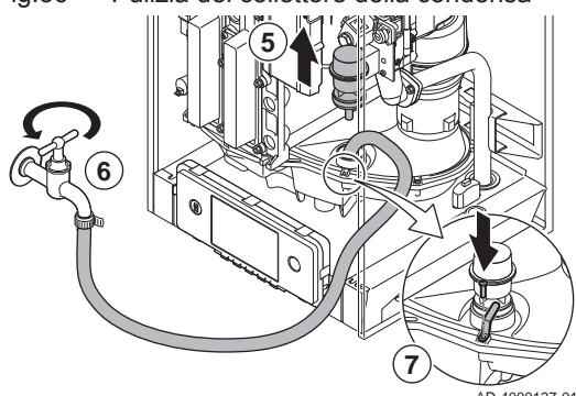
Fig.36 Pulizia del collettore della condensa
