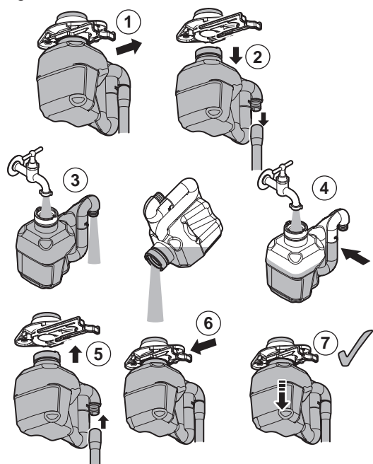
Fig.37 Pulizia del sifone
