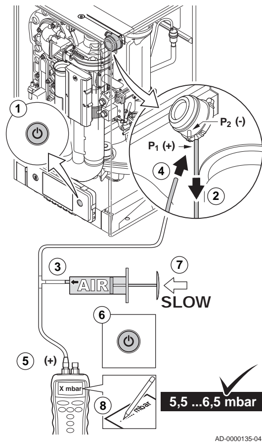
Fig.31 Controllare il pressostato differenziale lato +
