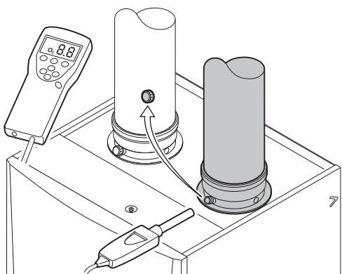
Fig.26 Presa analisi gas di scarico
