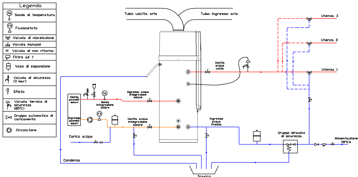
Schema di installazione in caso di ricircolo di acqua di integrazione solare Nota: il serpentino di integrazione solare è presente solo sui modelli LIBRA EASY SG
