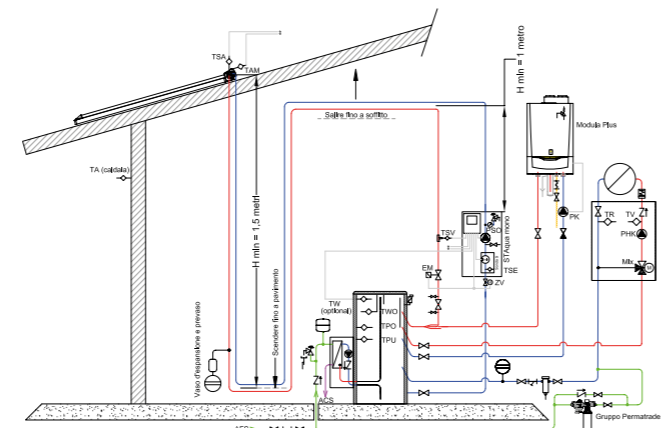
Impianto solare sottotetto con AQUA EXPRESSO III
