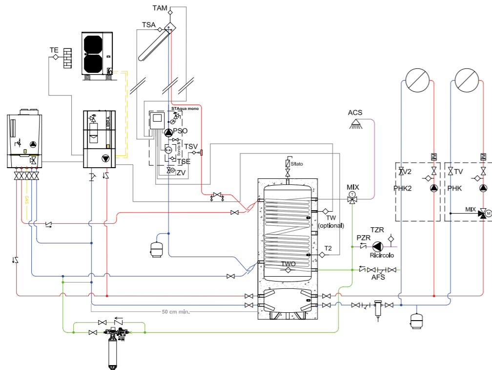
Pacchetti solari con bollitore RLH per produzione acqua calda sanitaria (THIT9456)
