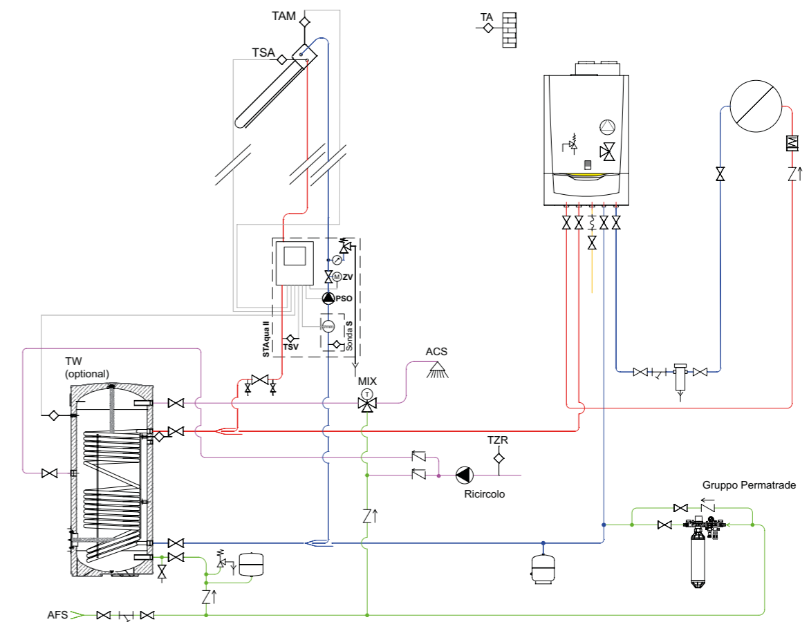
Pacchetti per bollitore monoserpentino, nel caso di pompa di carico bollitore e circuito diretto (THIT1767)
