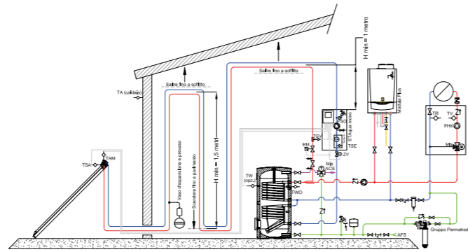
Impianto solare sottotetto con AquaSun Plus
