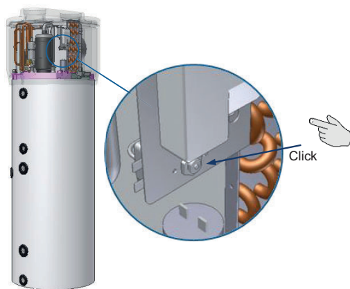
Fig. 17 – Ripristino termostato di sicurezza
