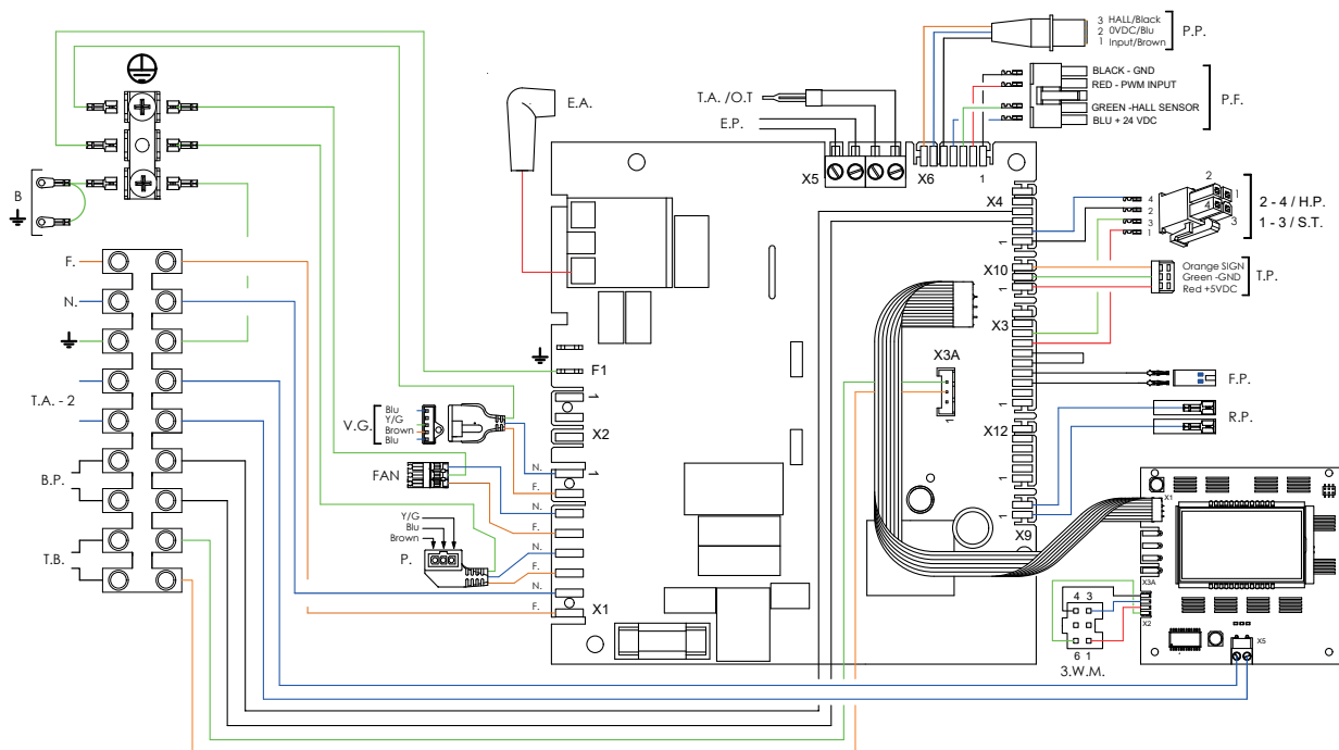
Legenda connessioni 3.W.M. Valvola Tre Vie F. Fase N. Neutro S.P. Sonda Sanitario T.B. Termostato Bollitore B. Terra Caldaia FAN Aspiratore fumi P. Circolatore S.T. Sonda Sicurezza V.G. Valvola Gas B.P. Sonda Bollitore FL. Flussostato P.F. PWM Ventilatore T.P. Trasduttore di Pressione E.A. Elettrodo Accensione F.P Sonda Fumi P.P. PWM Circolatore T.A./O.T Termostato Ambiente/Open Therm E.P. Sonda Esterna H.P. Sonda Riscaldamento R.P. Sensore Ritorno T.A. - 2 Termostato Ambiente Zona 2
